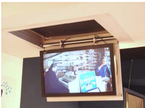
CMRD-L42 instalado y en posición de visionado.
