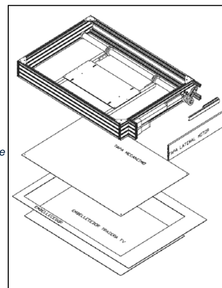
Layout despiece de soporte
